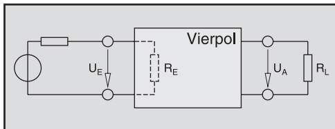
Bild 4 Die Leistungsverstärkung A_P des Vierpols kann in dB ausgedrückt werden.
