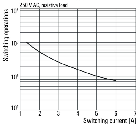
Elektrische Lebensdauer 230 V AC resistive load 230 V AC ohmsche Last
