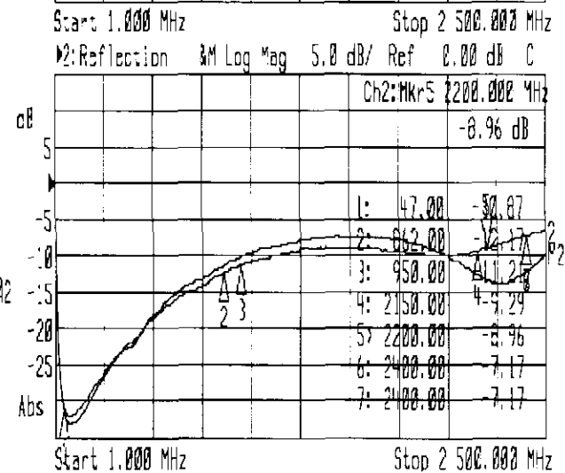
oben: Durchgangsdämpfung 20 dB unten: Rückflußdämpf. Eing./Ausg. bei 20 dB
