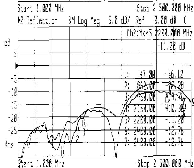
oben: Durchgangsdämpfung 0 dB unten: Rückflußdämpf. Eing./Ausg. bei 0 dB
