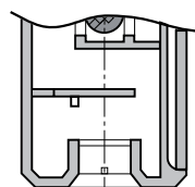
zwangsgeführte Zugentlastung
